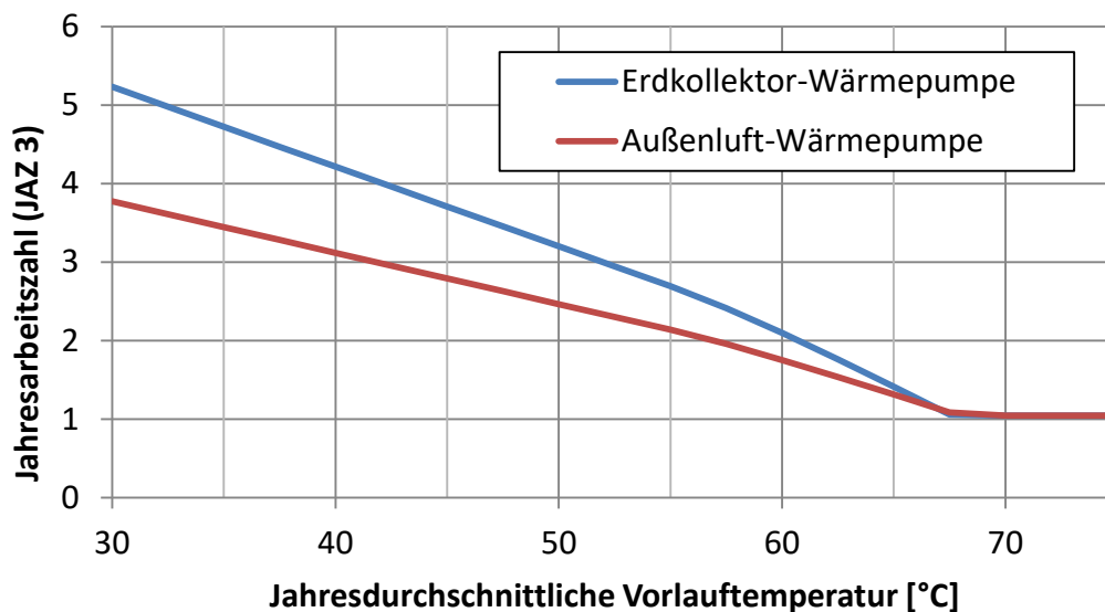
Abbildung 7: In den Berechnungen verwendeter Zusammenhang zwischen der Jahresarbeitszahl von Wärmepumpen und der durchschnittlichen Vorlauftemperatur des Wärmeverteilsystems
