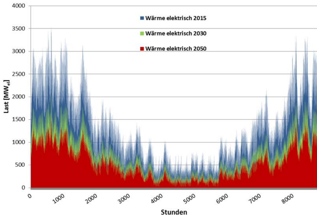
Abbildung 8: Strombedarf für die Wärmebereitstellung im Wärmewende Szenario für die Jahre 2015, 2030 und 2050
