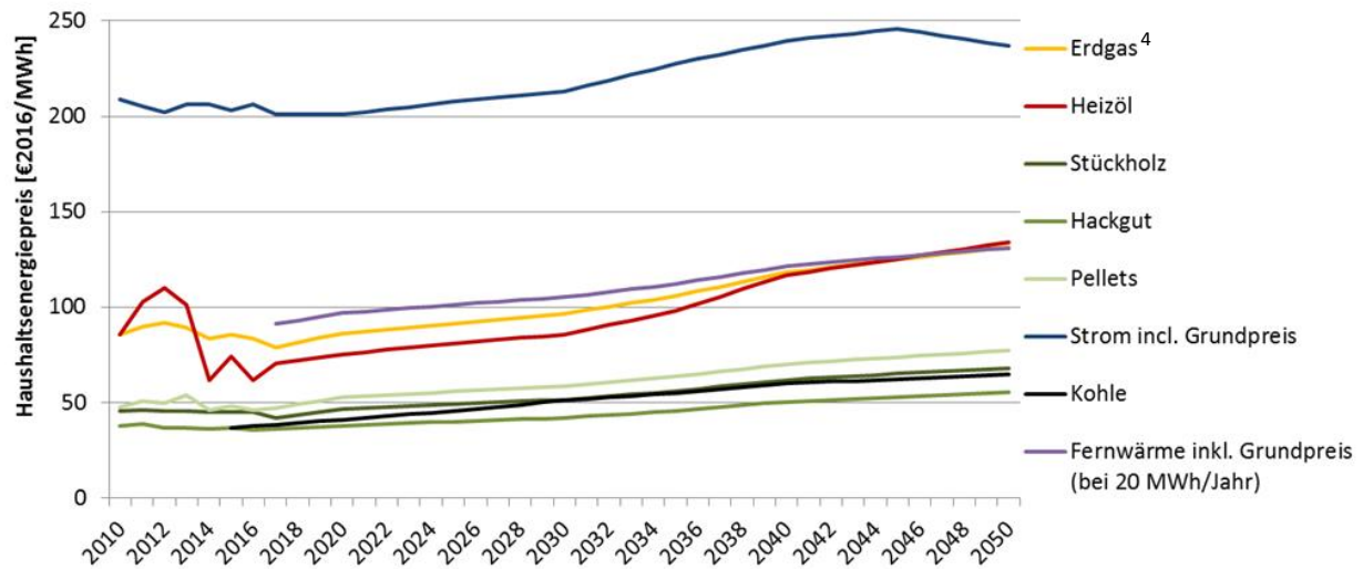
Abbildung 12: Angenommene jährliche Energiekosten der Heizsysteme (Empfehlung der EU Kommission)
