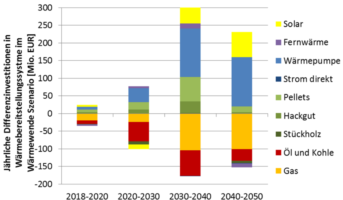
Abbildung 10: Jährliche Differenzinvestitionen in Wärmebereitstellungssysteme im Wärmewende Szenario gegenüber Referenzszenario
