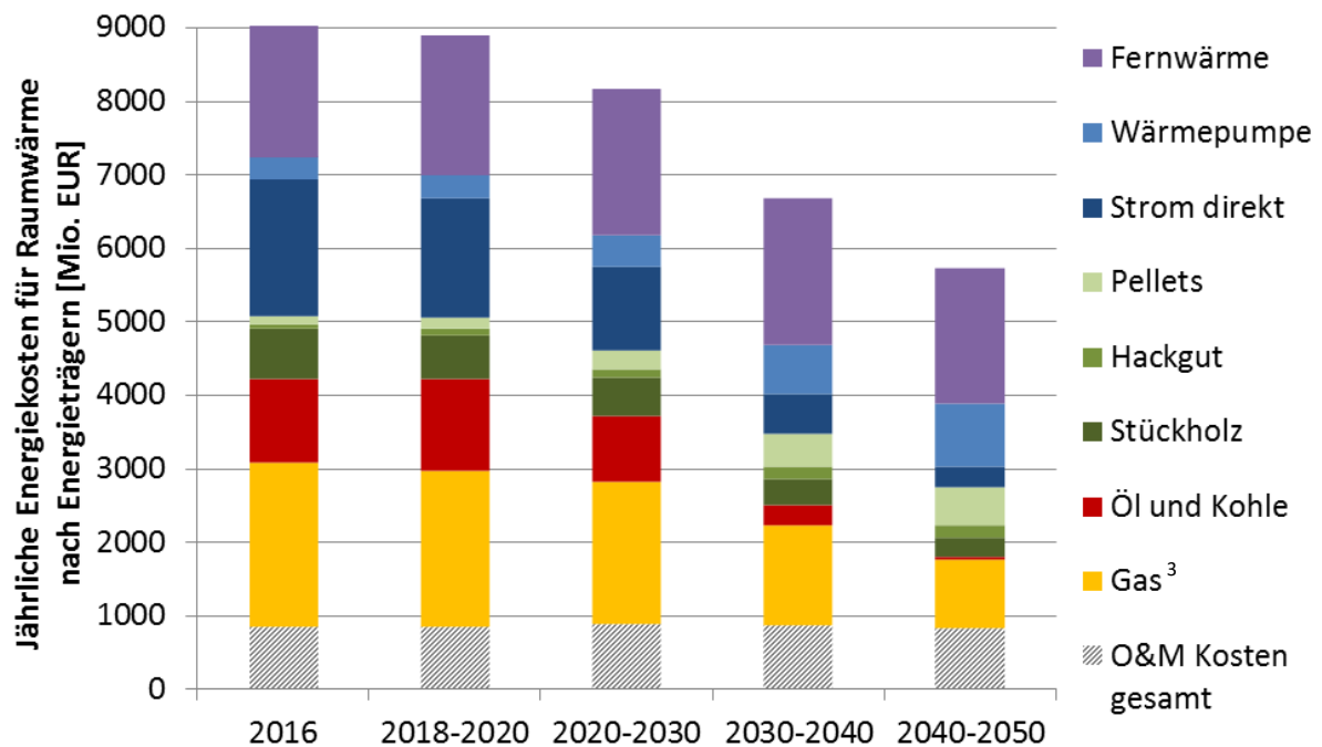
Abbildung 11: jährliche Energiekosten der Heizsysteme im Wärmewende Szenario 3
