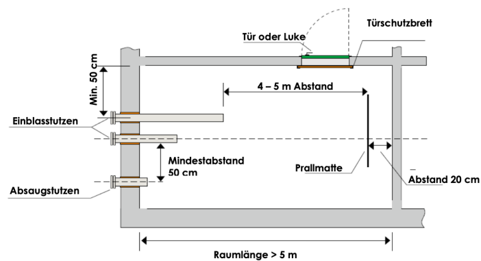
Bild 3 – Grundriss eines Pelletslagerhauses (Belüftung über Befüllsystem)
